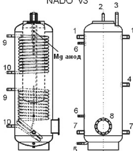
NADO v3
