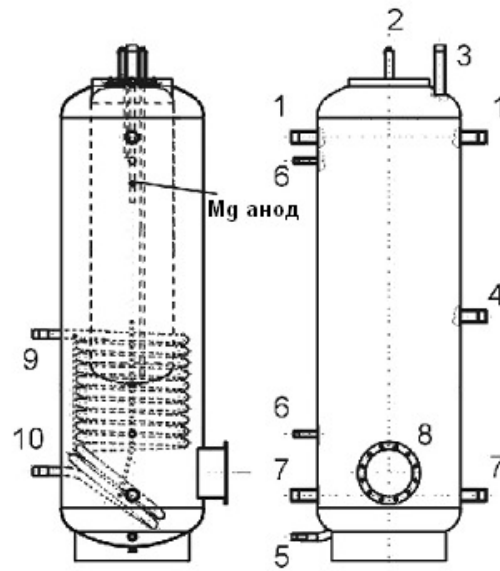
NADO v2
