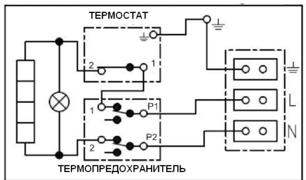
СХЕМА ЭЛЕКТРИЧЕСКОГО ПОДКЛЮЧЕНИЯ С ТЕРМОСТАТОМ «EICA v01» И ТЕРМОПРЕДОХРАНИТЕЛЕМ «EICA mag01»
