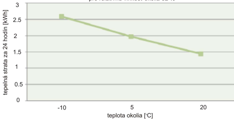
Tepelná strata vonkajšej nádrže NAD 500 v8 pre relatívnu vlhkosť okolia 52 %
