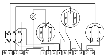
SCHEMA ELEKTRICKÉHO ZAPOJENÍ PRO 3 - 6 kW
