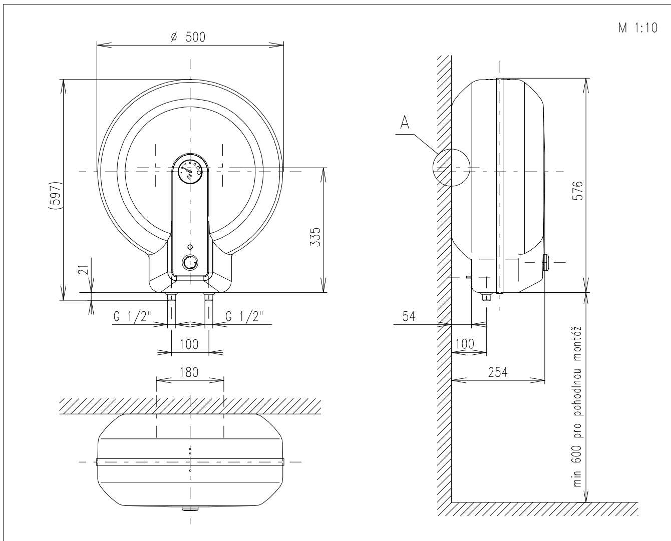
obrázek 1: ROZMĚRY
