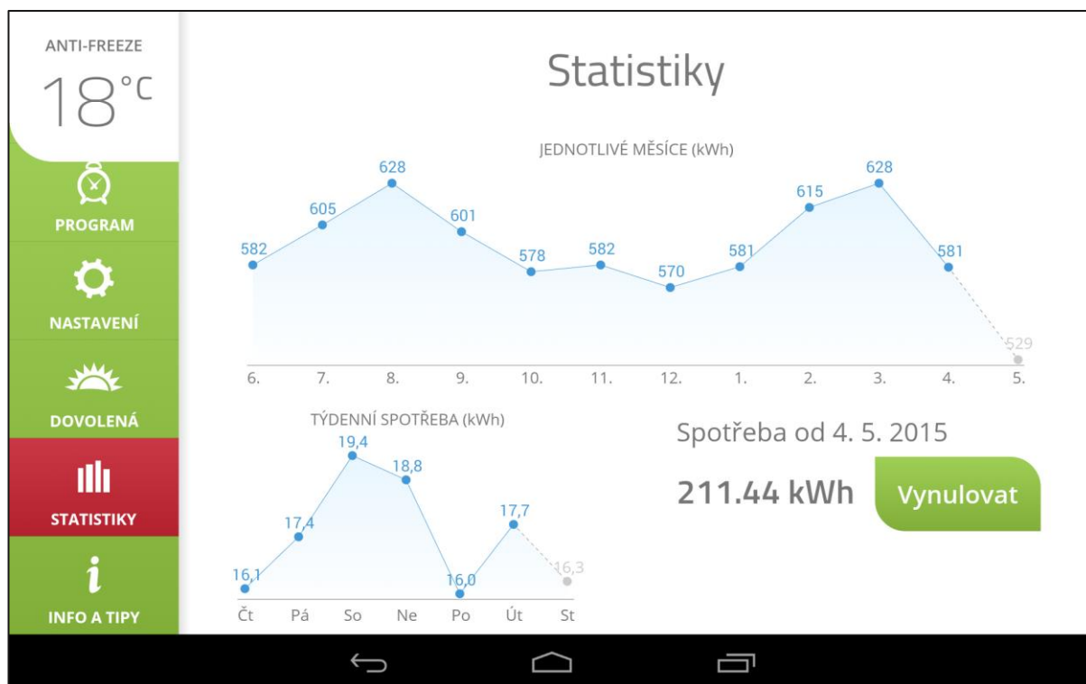
Obrázek 16: Obrazovka Statistiky
