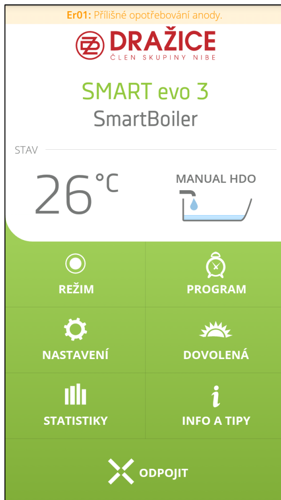
Obrázek 10: Navigační panel
