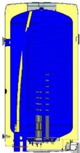
Řez kombinovaným zásobníkem OKHE 125 NTR/DV
