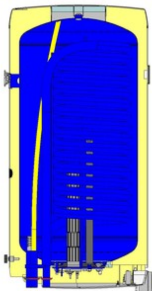
Řez kombinovaným zásobníkem OKHE 125 NTR/DV
