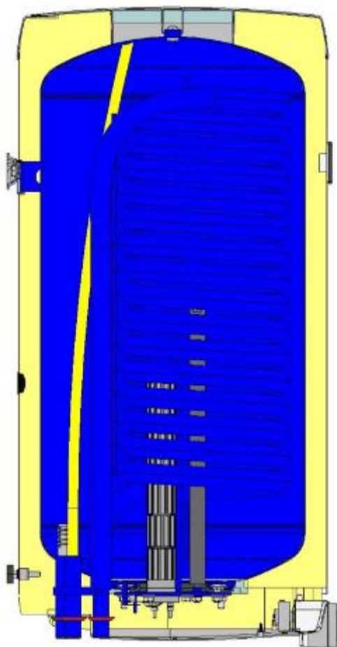
Řez kombinovaným zásobníkem OKHE 125 NTR/DV
