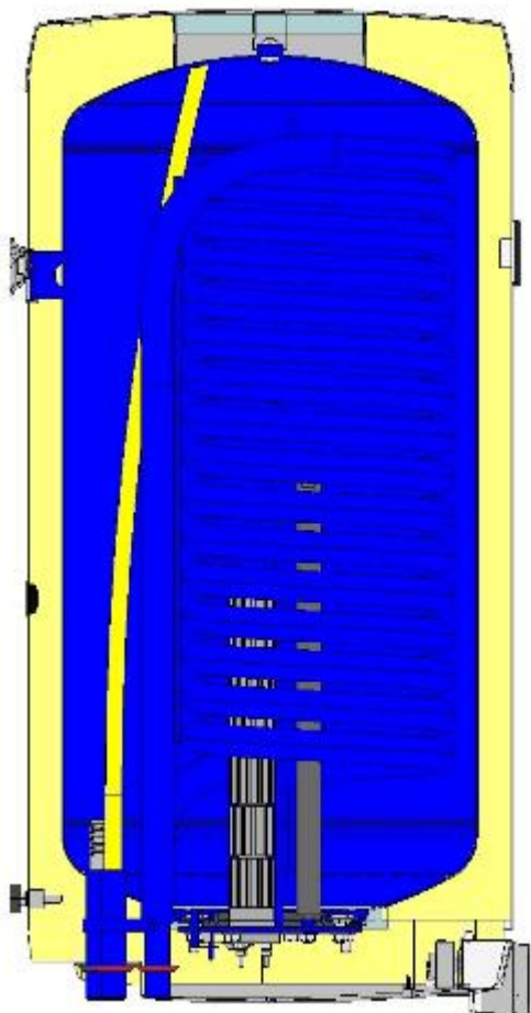
Řez kombinovým zásobníkem OKHE 125 NTR/DV
