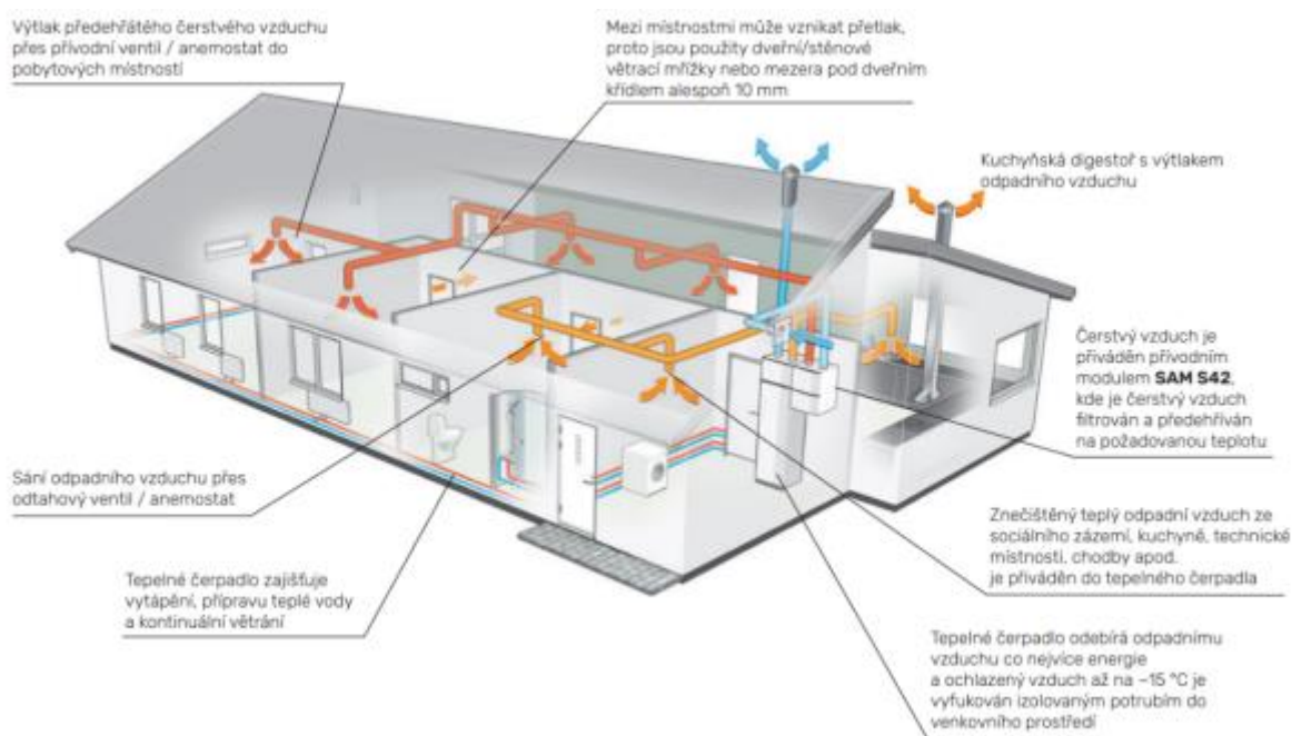
Tepelné čerpadlo systému vzduch-voda NIBE S2125 (obr. 1)
