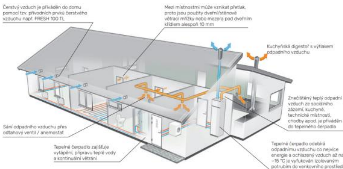
Tepelné čerpadlo systému vzduch-voda NIBE S2125 (obr. 2)
