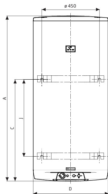
Horní a spodní závěs 160, 180, 200 l 4 kotevní šrouby
