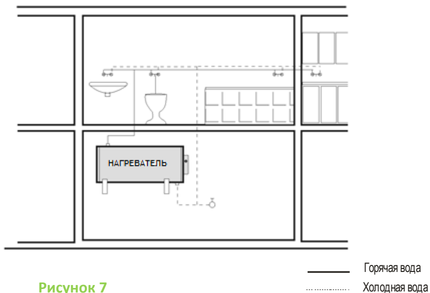
АККУМУЛИРУЮЩИЙ ВОДОНАГРЕВАТЕЛЬ ЭЛЕКТРИЧЕСКИЙ РАСПРЕДЕЛИТЕЛЬНАЯ СЕТЬ ГОРЯЧЕЙ ВОДЫ
