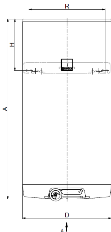
Верхний подвес 50-160 л 2 анкерных винта
