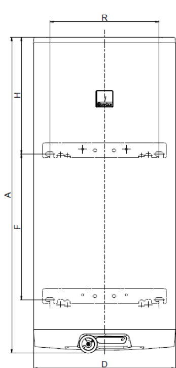
Верхний и нижний подвес 200 л 4 анкерных винта Размеры 450 мм и F Перед сверлением проверить
