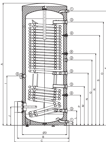
ОКС 500 NTRR/HP/SOL
