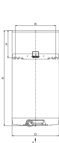
ОКСЕ 125-160 2/2 кВт
