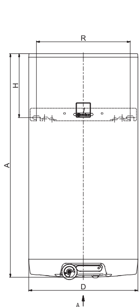
ОКСЕ 125–160 2/6 кВт
