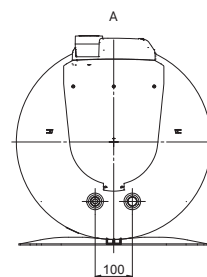
ОКСЕ 125-160 2/2 кВт
