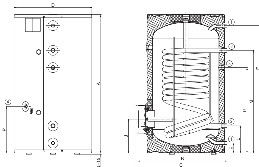
OKS 160 NTR/BP
