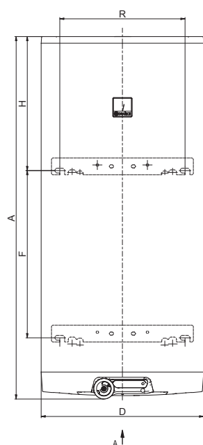
ОКСЕ 200 2/6 кВт
