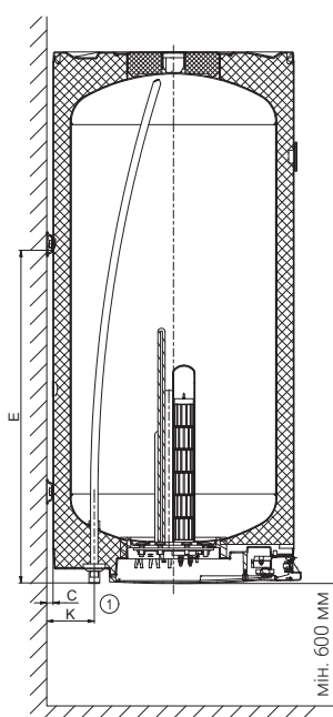
ОКСЕ 200 2/2 (4) кВт
