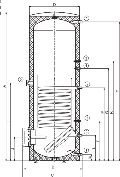
OKS 500 NTR/BP
