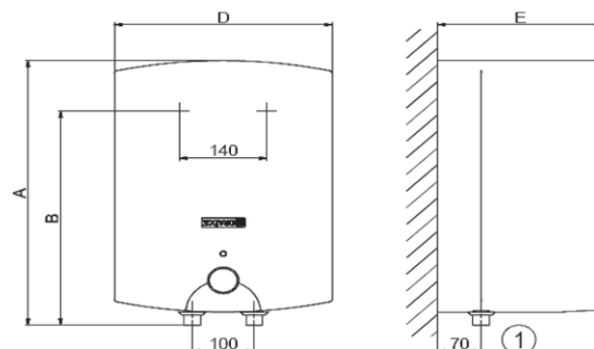
ВТО 10 UP
