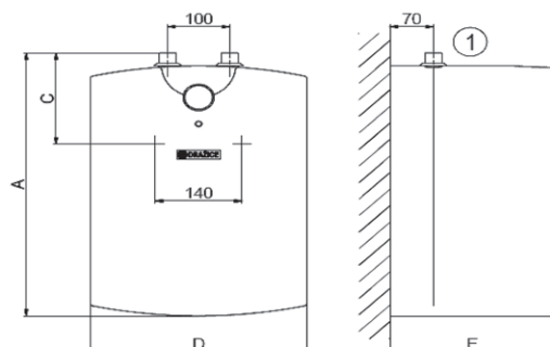
ВТО 10 IN
