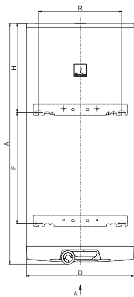
ОКСЕ 200 2/2 (4) кВт
