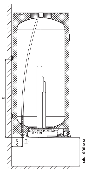
ОКСЕ 200 2/6 кВт
