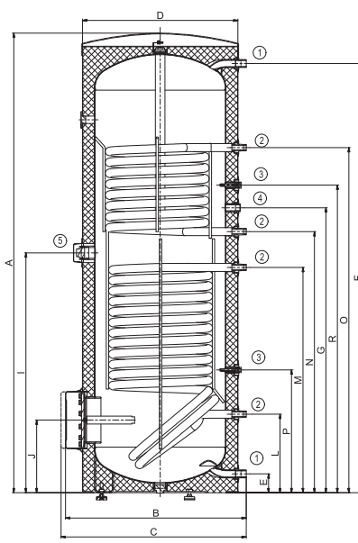
OKS 500 NTRR/BP
