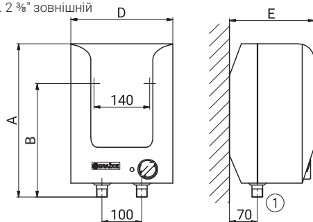
ВТО 5 UP
