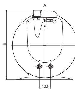
ОКСЕ 200 2/2 (4) кВт
